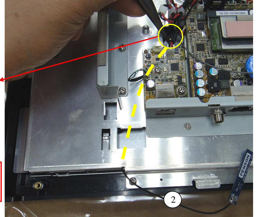
RFID天線LCD BRACKET底穿進，由SPEAKER孔位穿出，需用尖嘴夾子取出天線。
