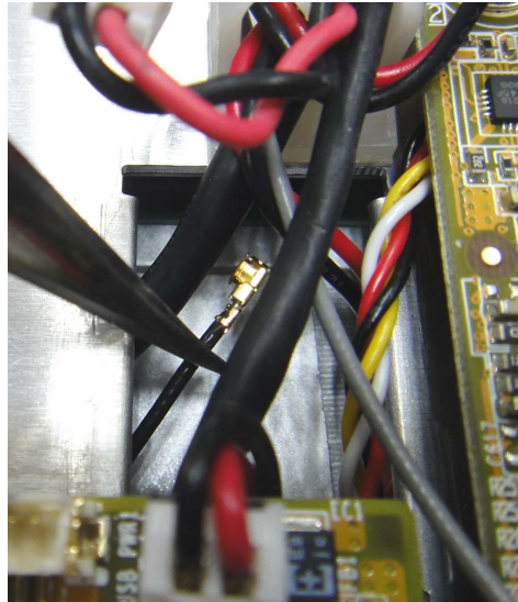
RFID天線LCD BRACKET底穿進，由SPEAKER孔位穿出，需用尖嘴夾子取出天線。
